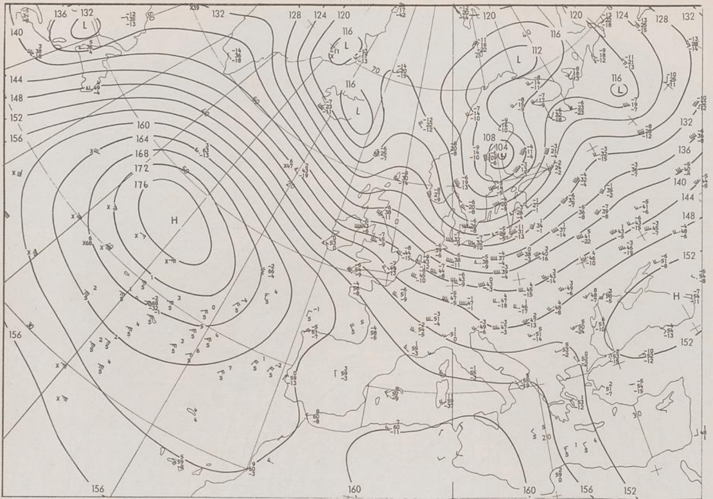
850 mbar 00 GMT
