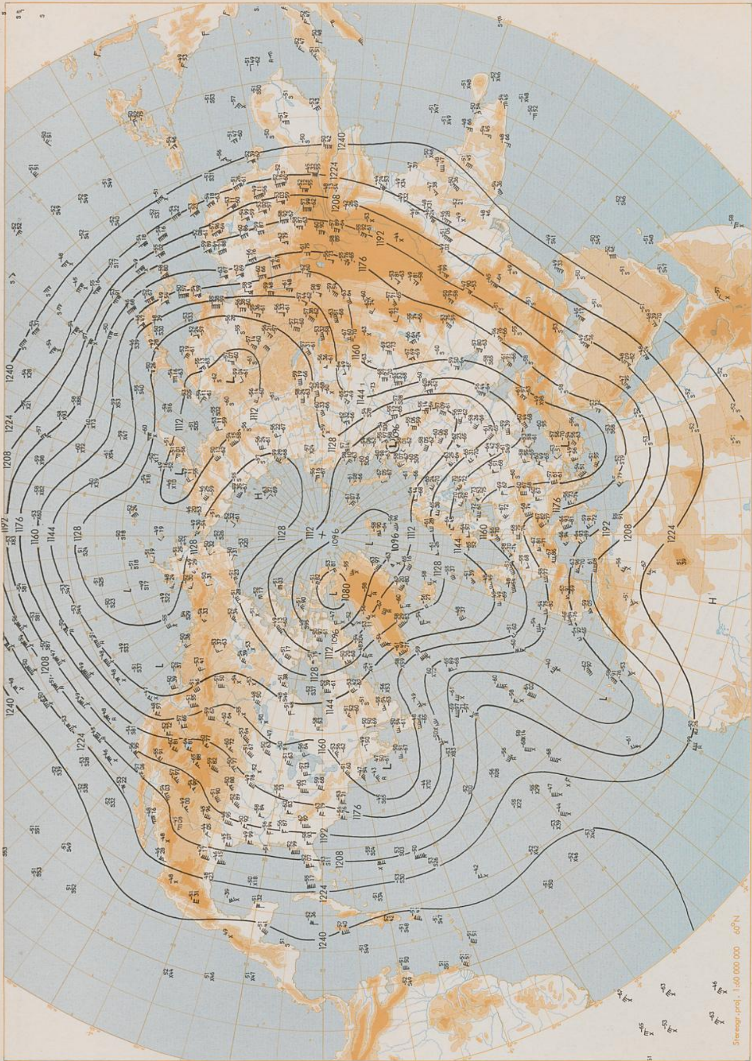
200 mbar ○○ GMT
