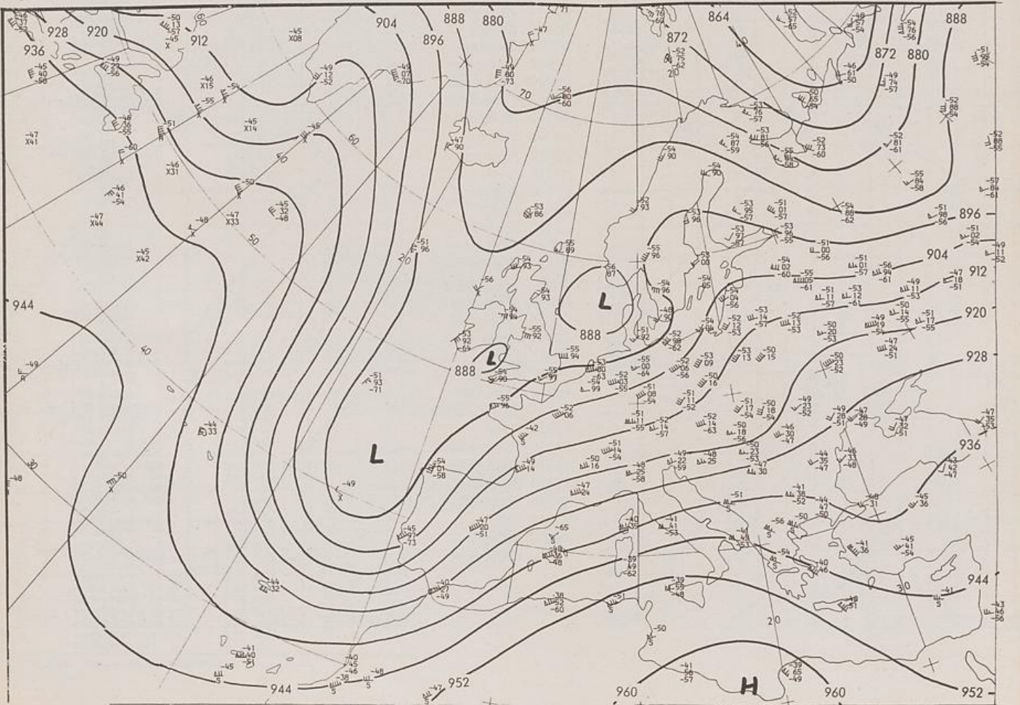
300 mbar 00 GMT
