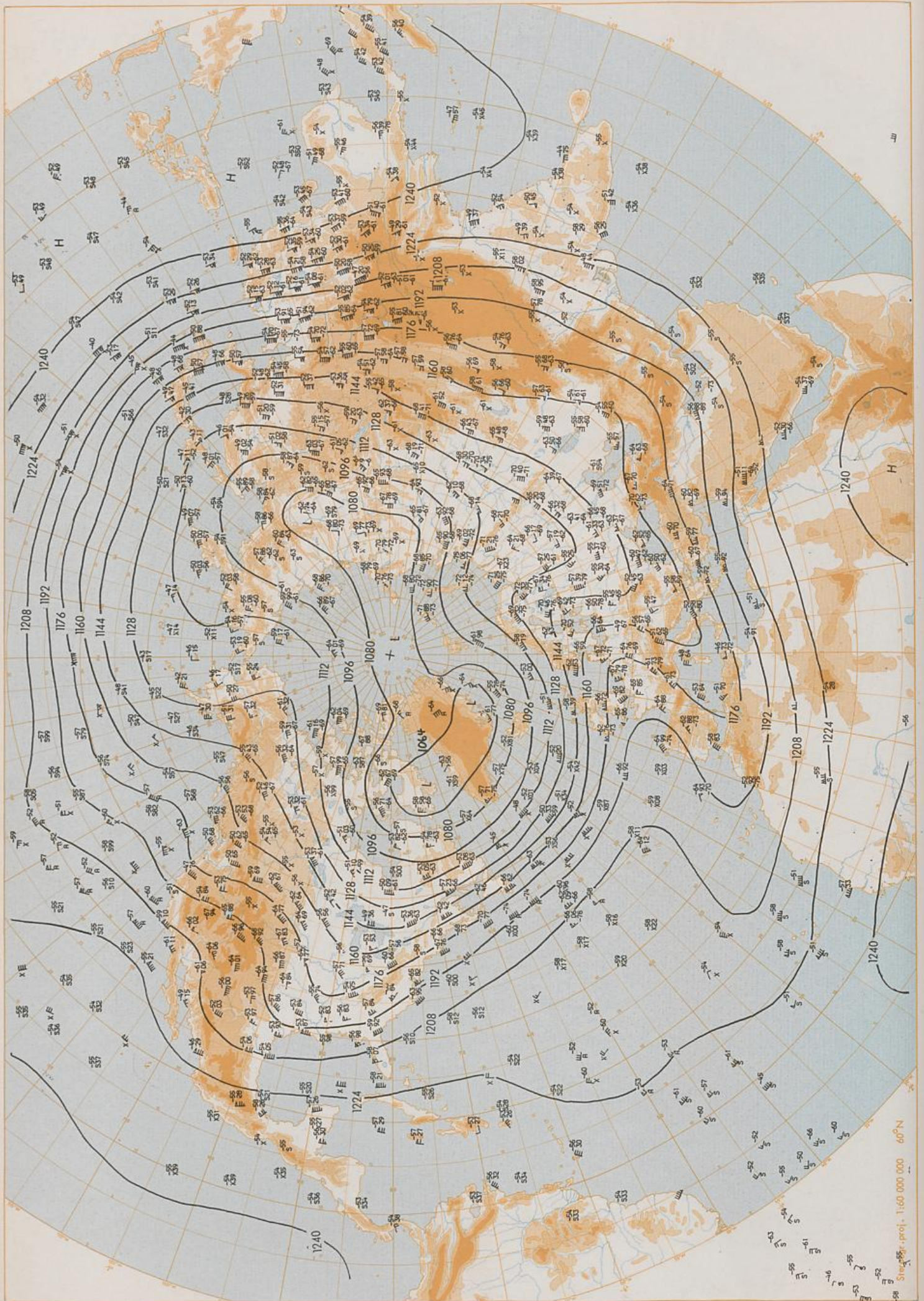
200 hPa 00 GMT
