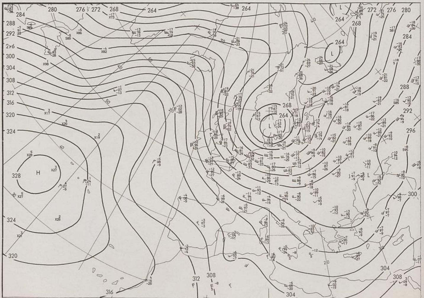
700 hPa 00 GMT
