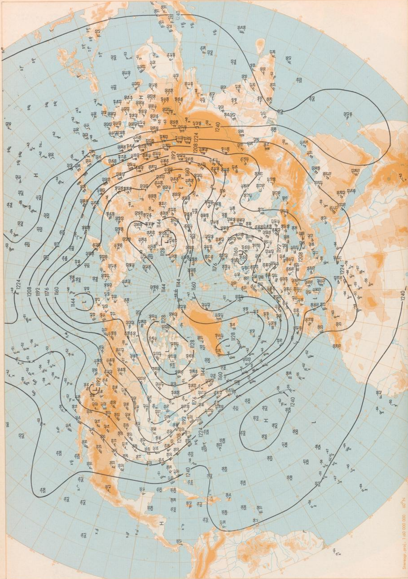
200 hPa 00 GMT
