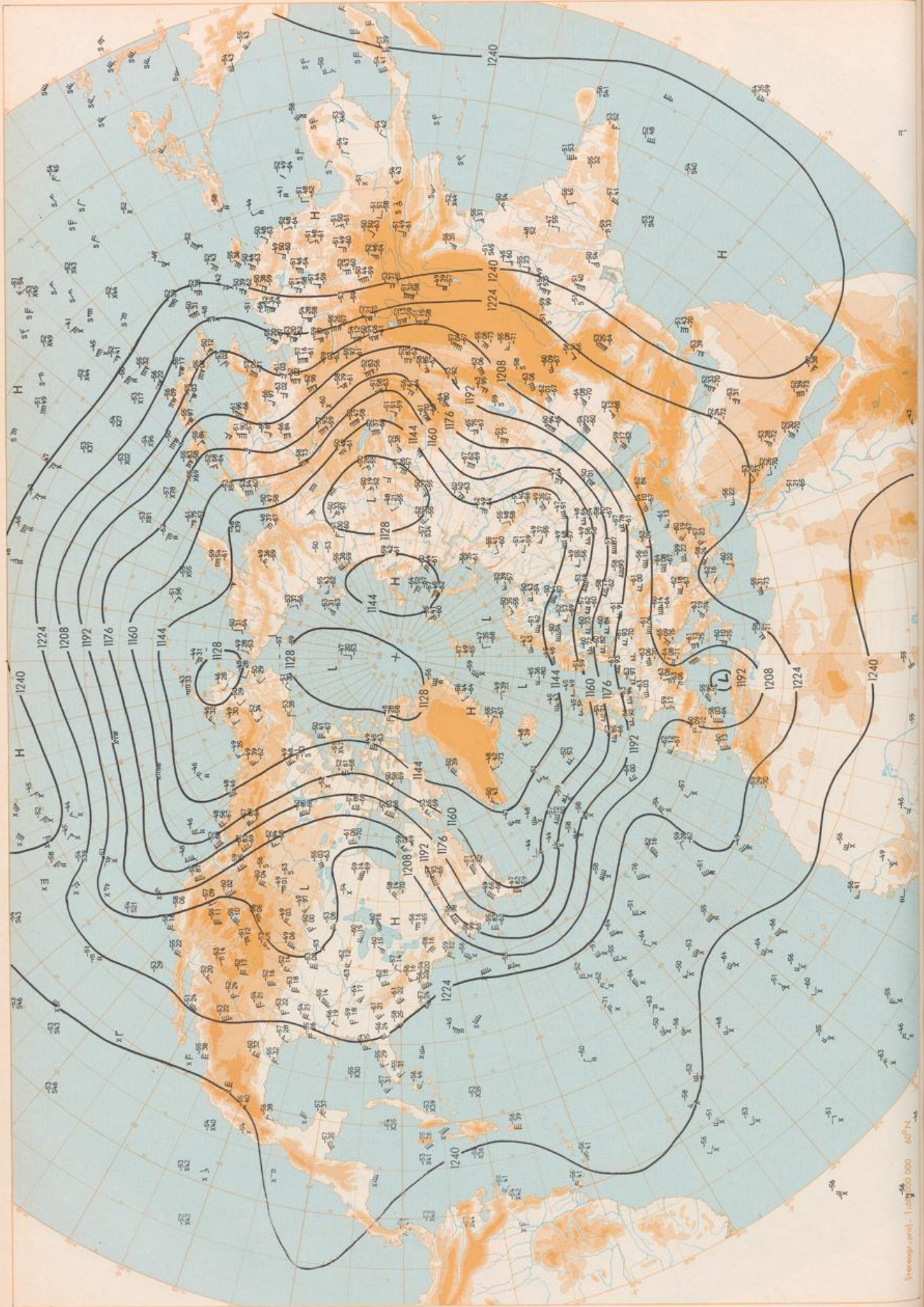
200 hPa 00 GMT
