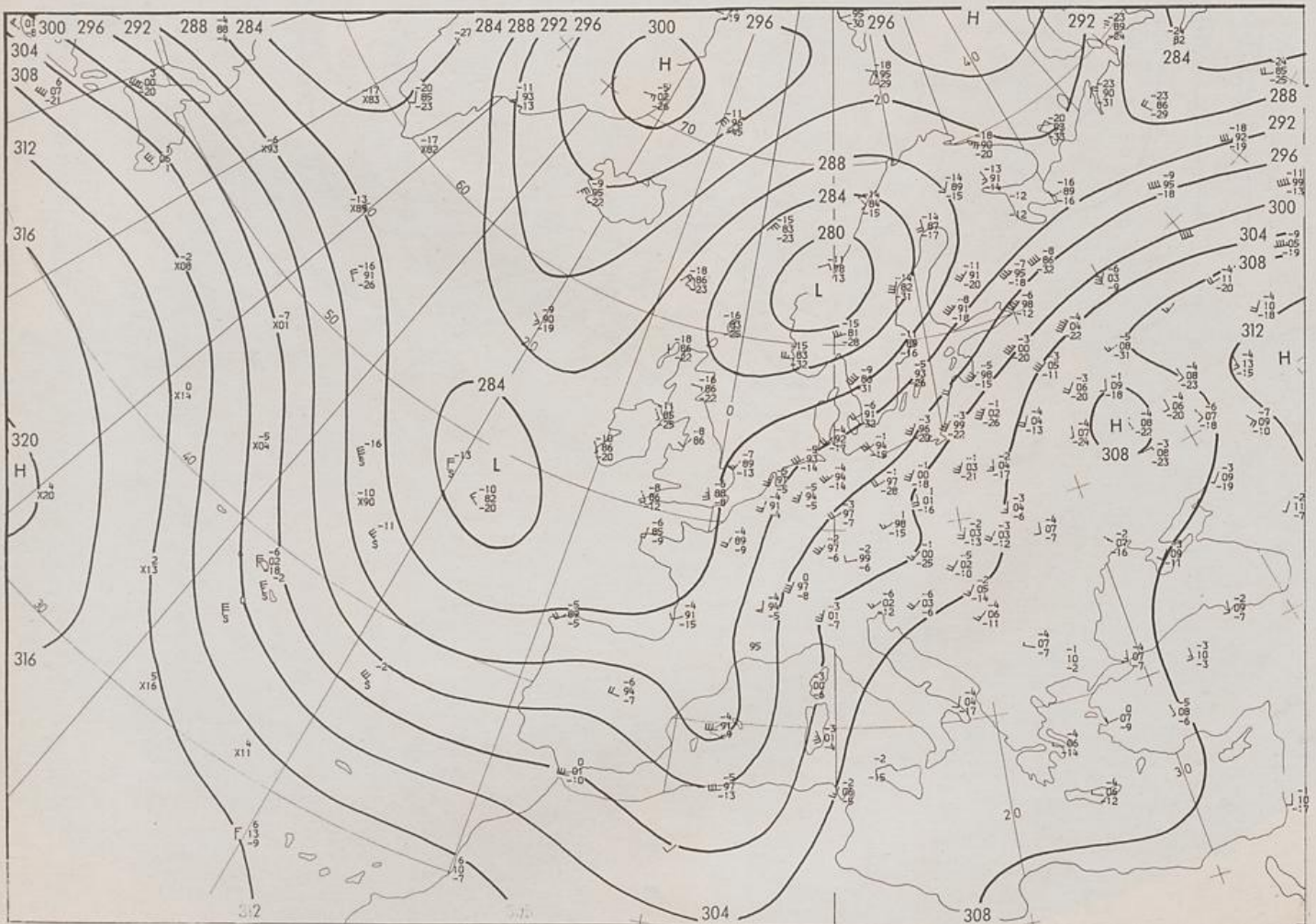
700 hPa 00 GMT
