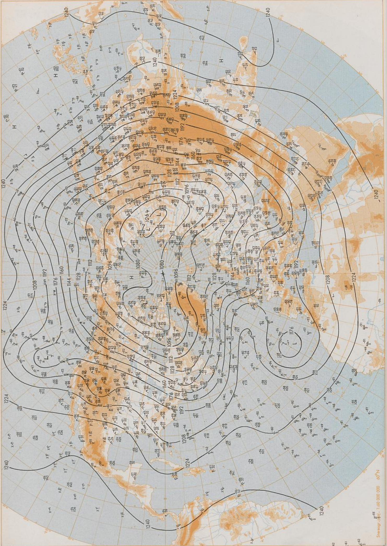
200 hPa 00 GMT
