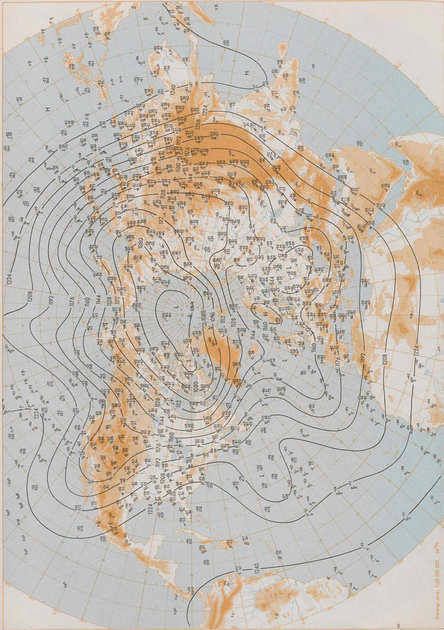
200 hPa 00 GMT
