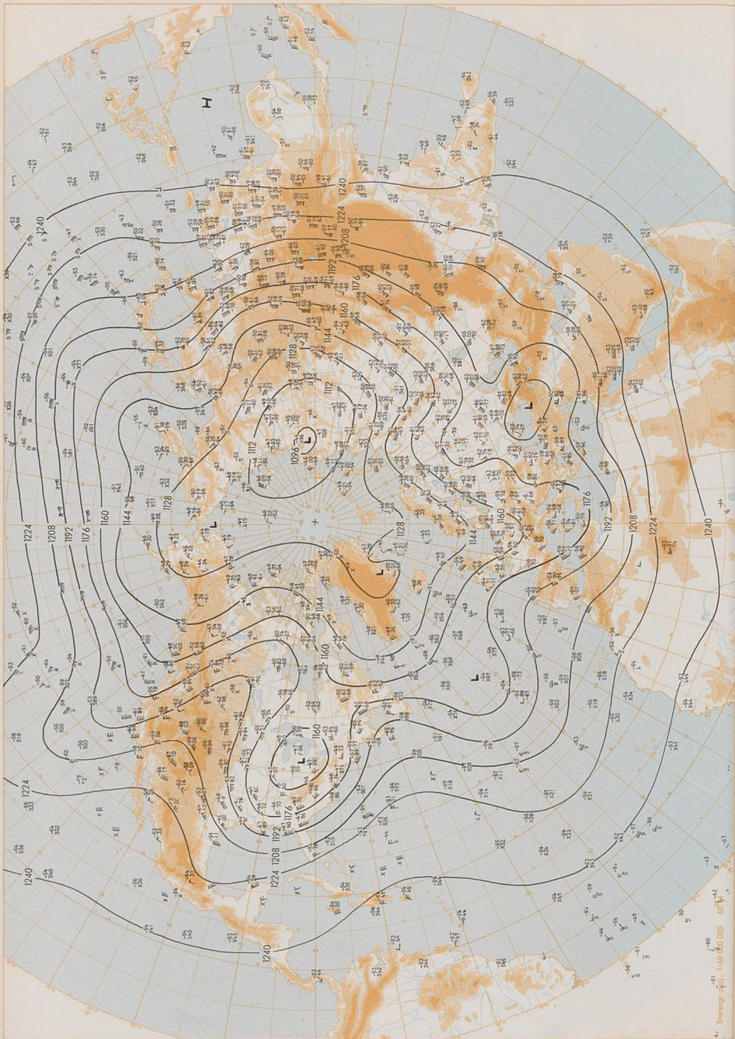
200 hPa 00 GMT
