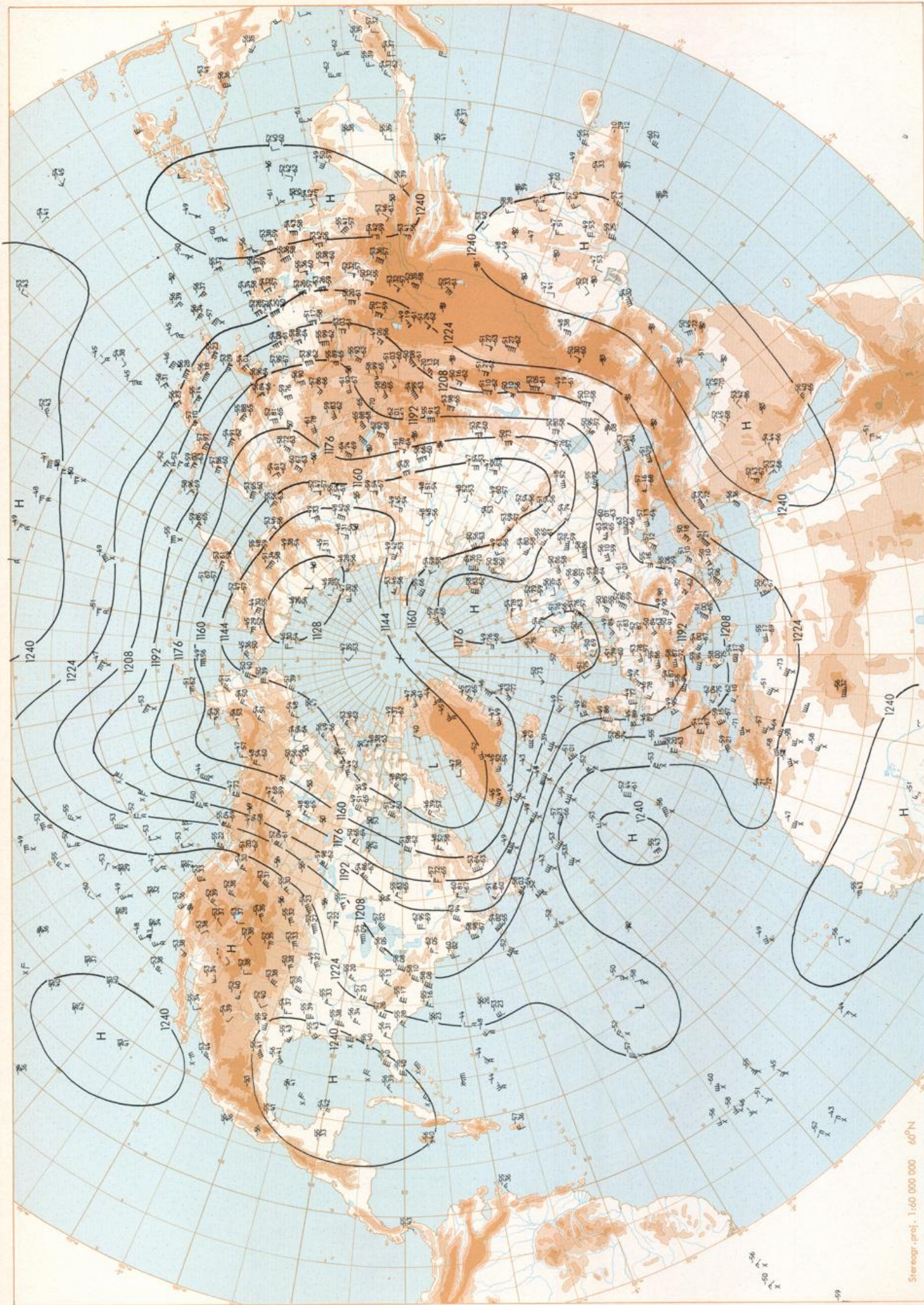
200 hPa 00 GMT
