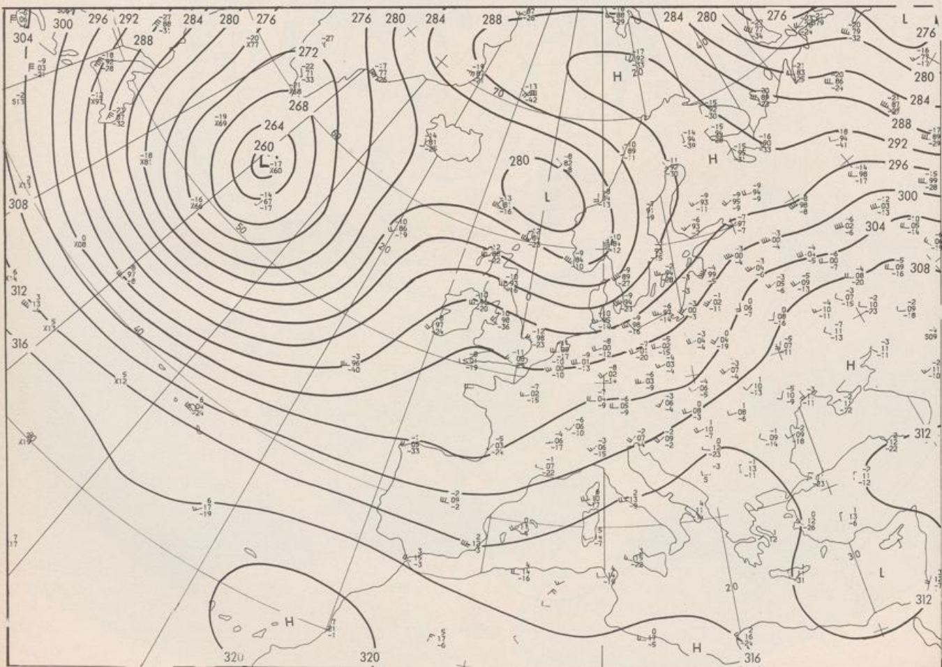
700 hPa 00 GMT
