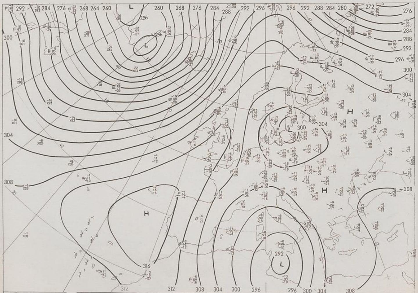
700 hPa 00 GMT
