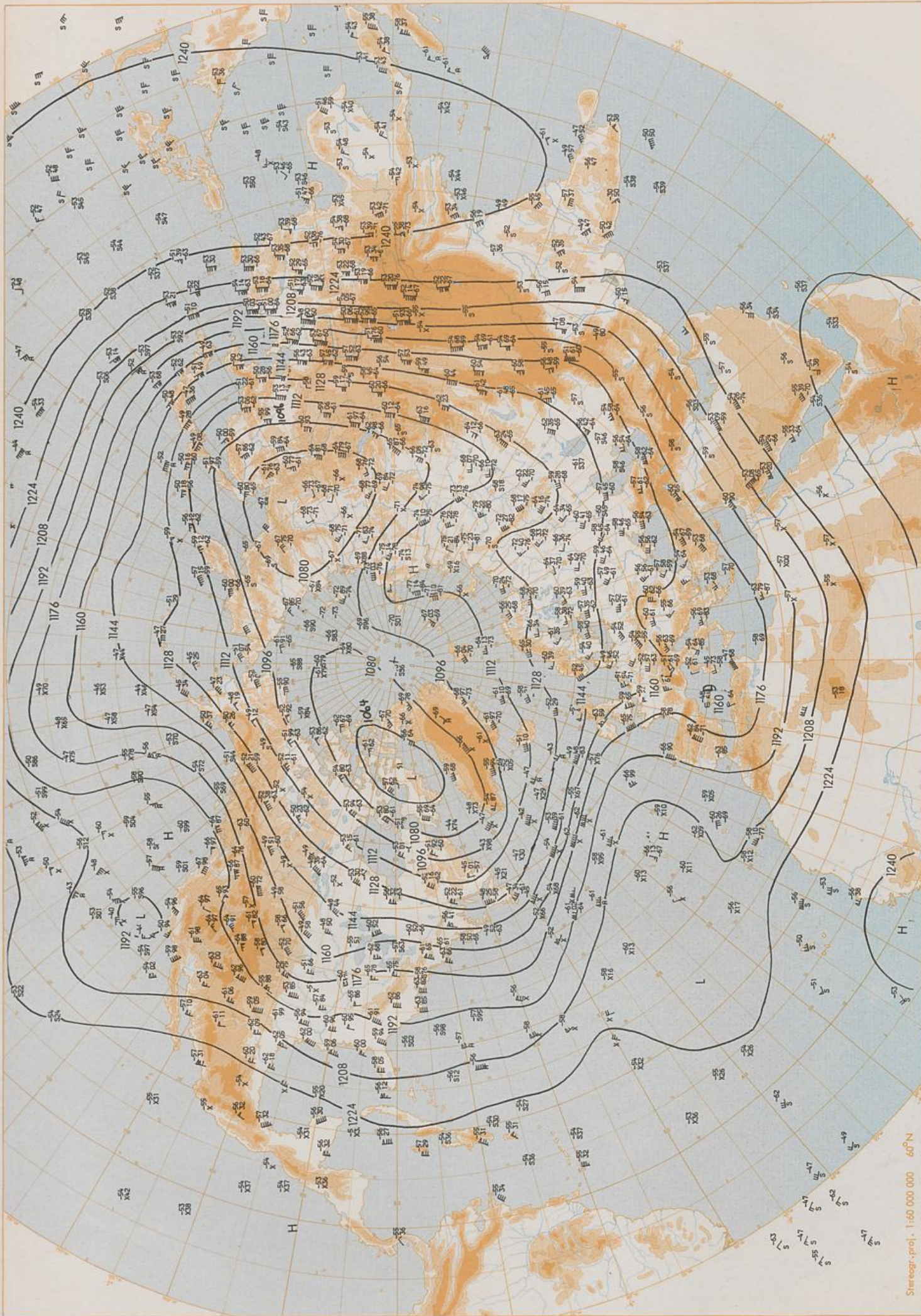
200 hPa 00 GMT
