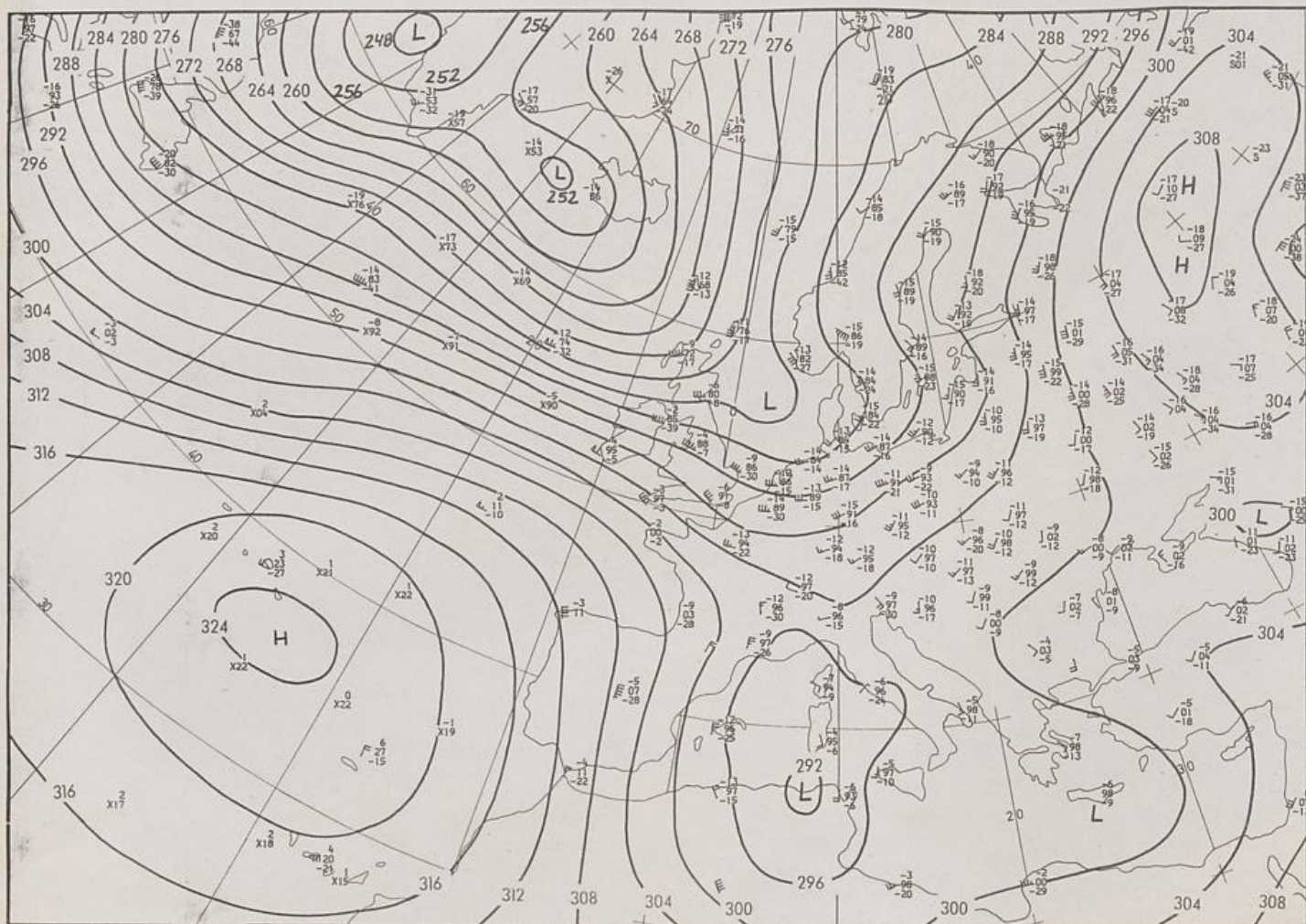
700 hPa 00 GMT
