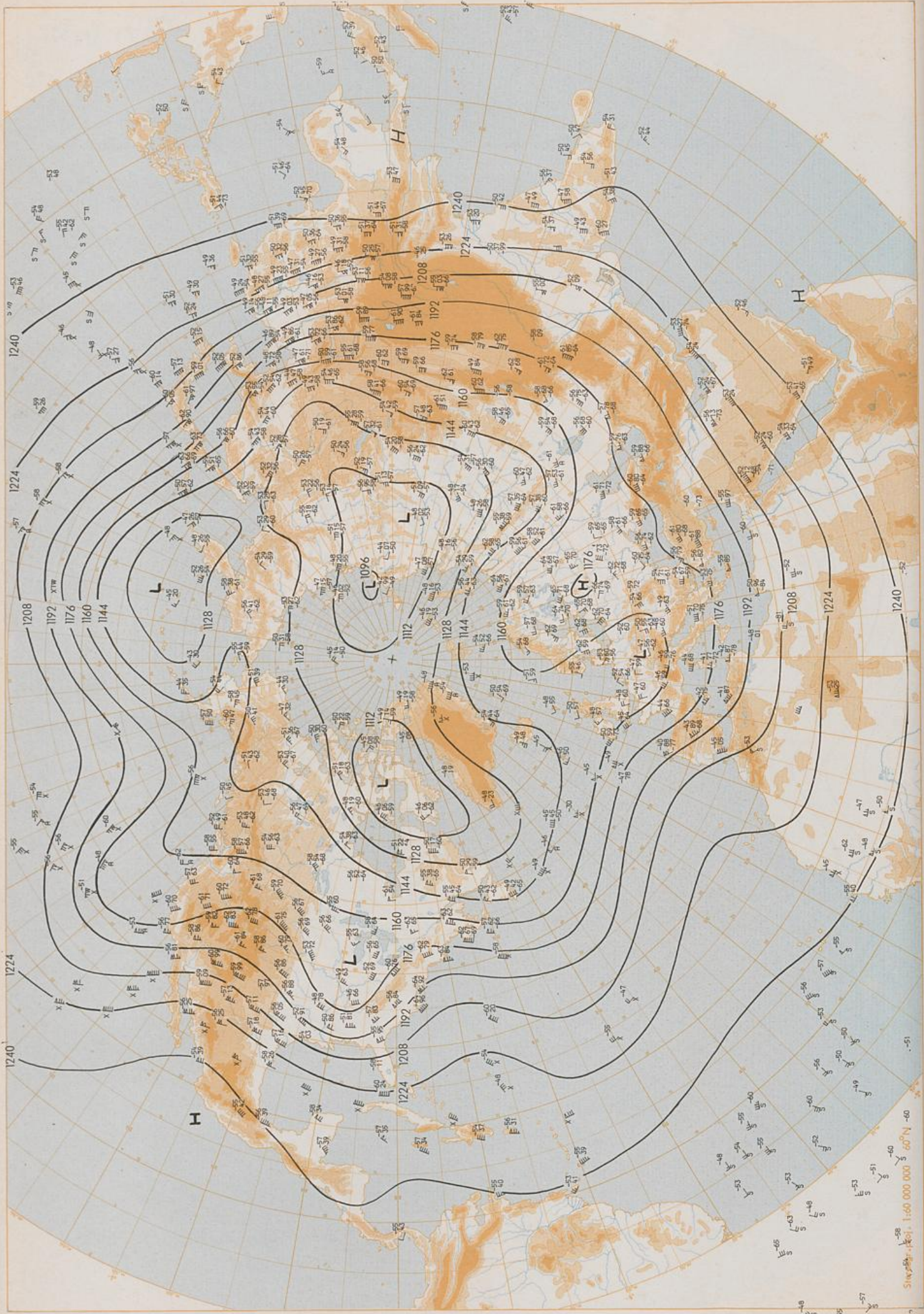
200 hPa 00 GMT
