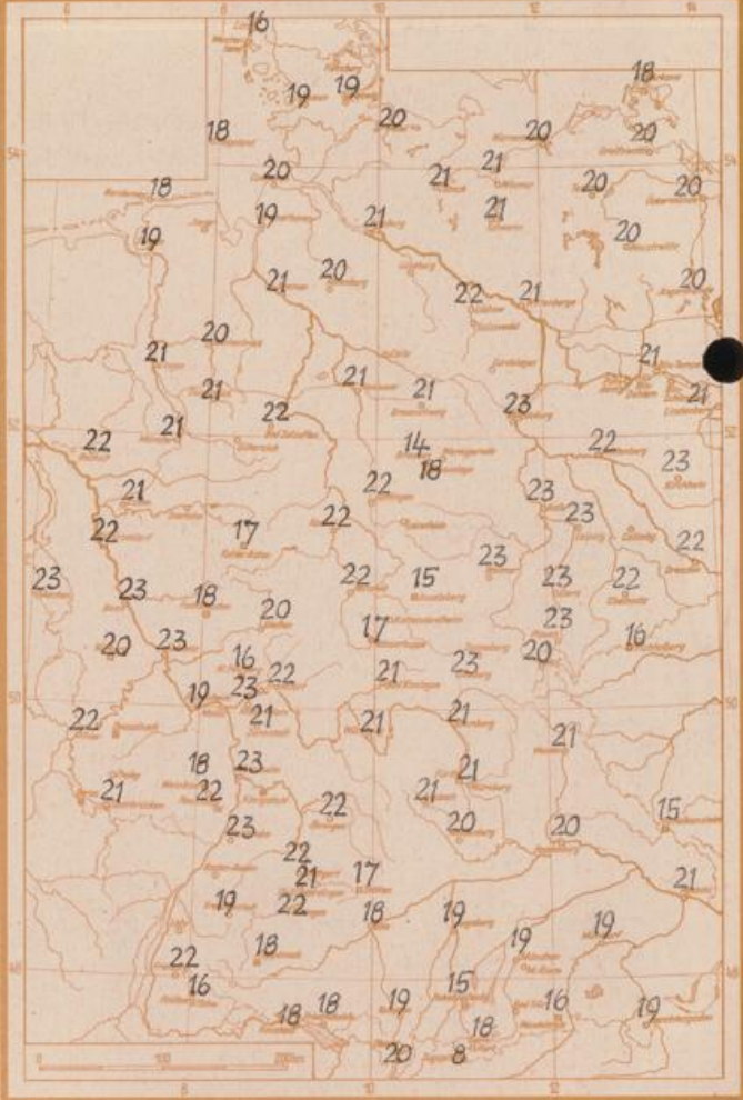
Höchsttemperaturen am 10.10.61 in 2 m Höhe in Grad C
