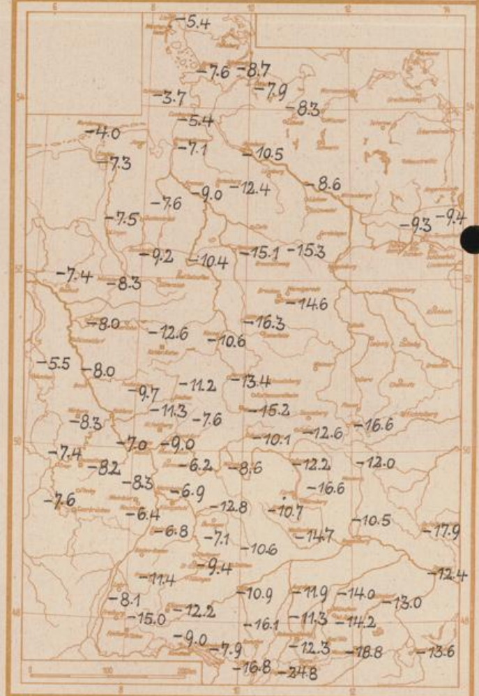
Tiefste Lufttemperaturen im März 1962 in 2 m Höhe in Grad C
