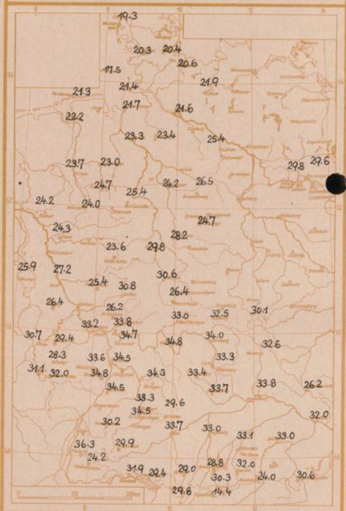
Höchste Lufttemperaturen im August 1962 in 2 m Höhe in Grad C
