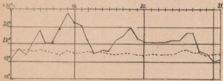
Tagesmitteltemperaturen Juli 1959 in Essen
