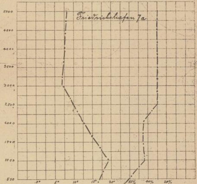
Zustandskurven heute morgen, Temp. in Grad. C. Höhe %.
