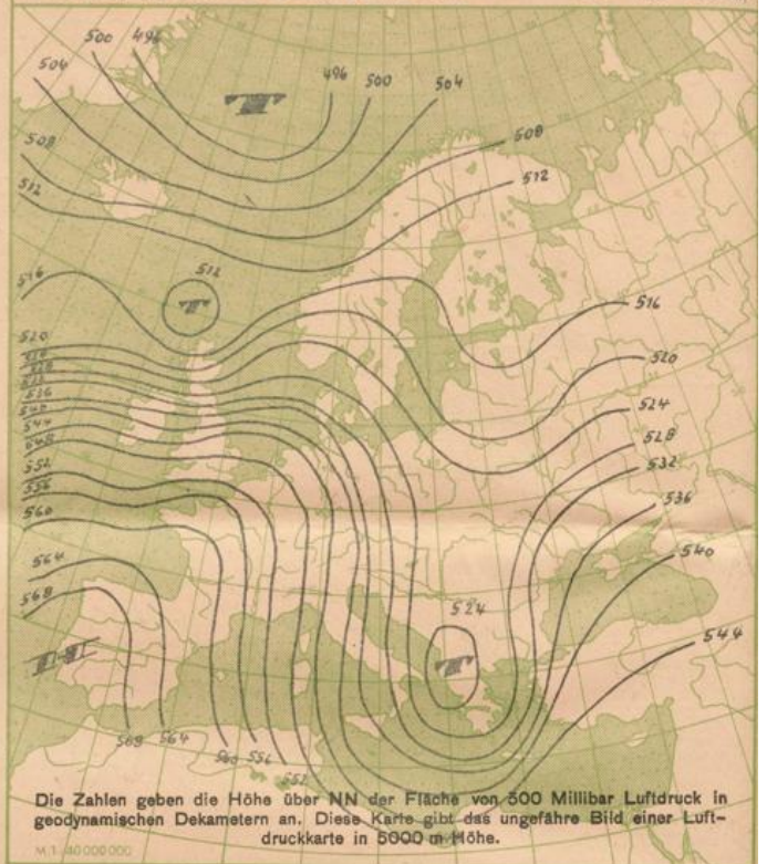
Absol. Topographie der 500 mb Fläche vom 2. 1. 1948 00 00 MGZ
