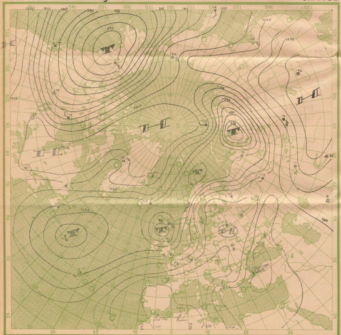
Wetterkarte der Nordhalbkugel vom 1. Januar 1948
