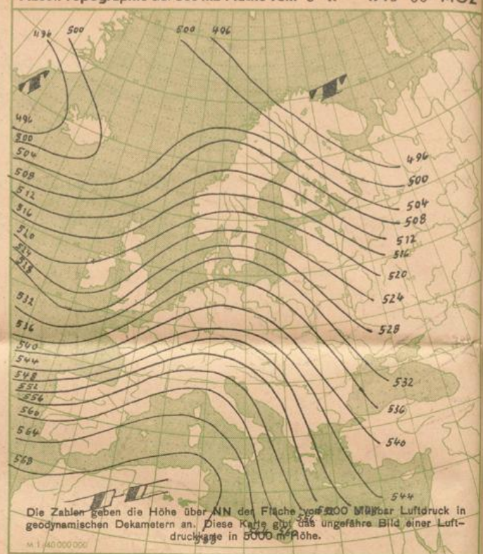
Wetterkarte der Nordhalbkugel vom 4. Januar 1948 18 00 Uhr MGZ
