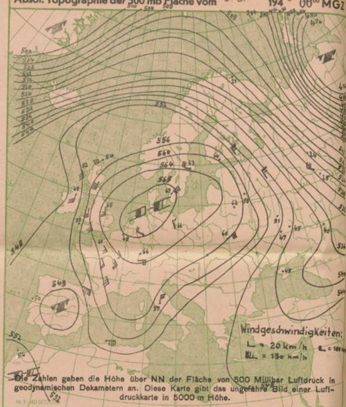
Absol. Topographie der 500 mb Fläche vom 5. 3. 1948 00 00 MGZ
