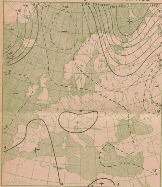
Wetterkarte der Nordhalbkugel vom 4. März
