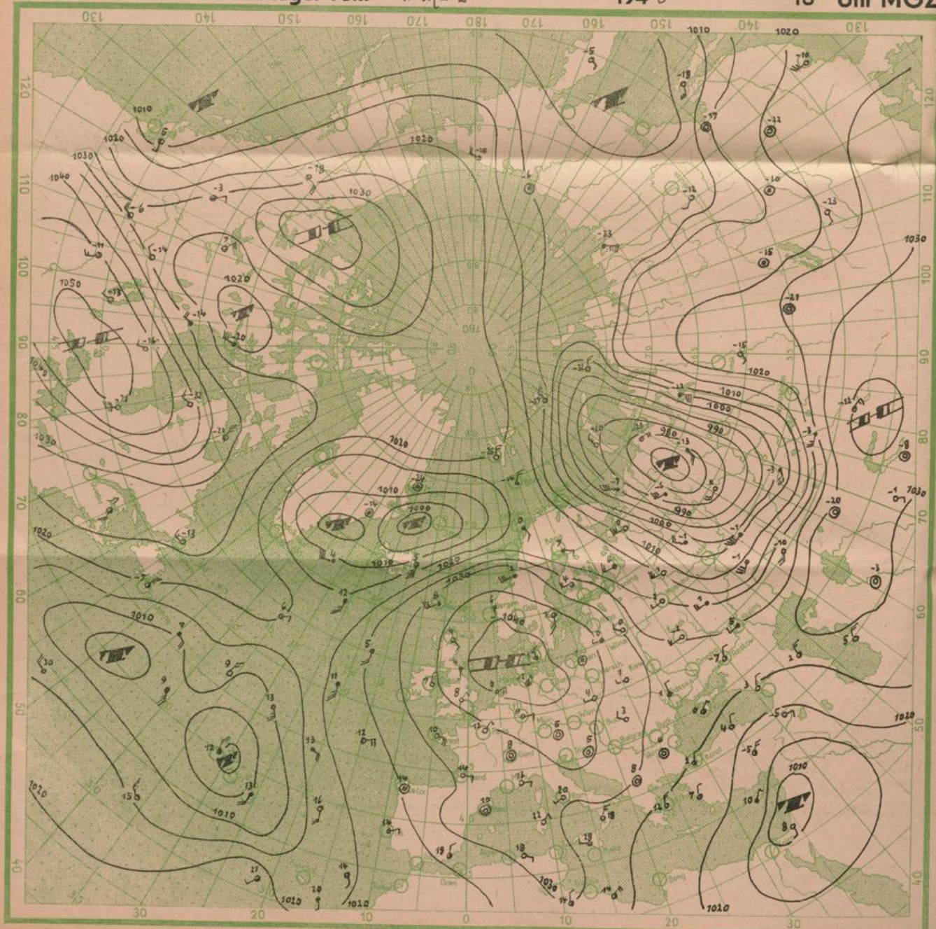
Wetterkarte der Nordhalbkugel vom 4. März
