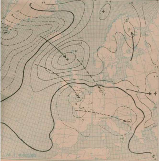
Luftdruckänderung seit gestern 8 Uhr (2,5 Stg. mb)
