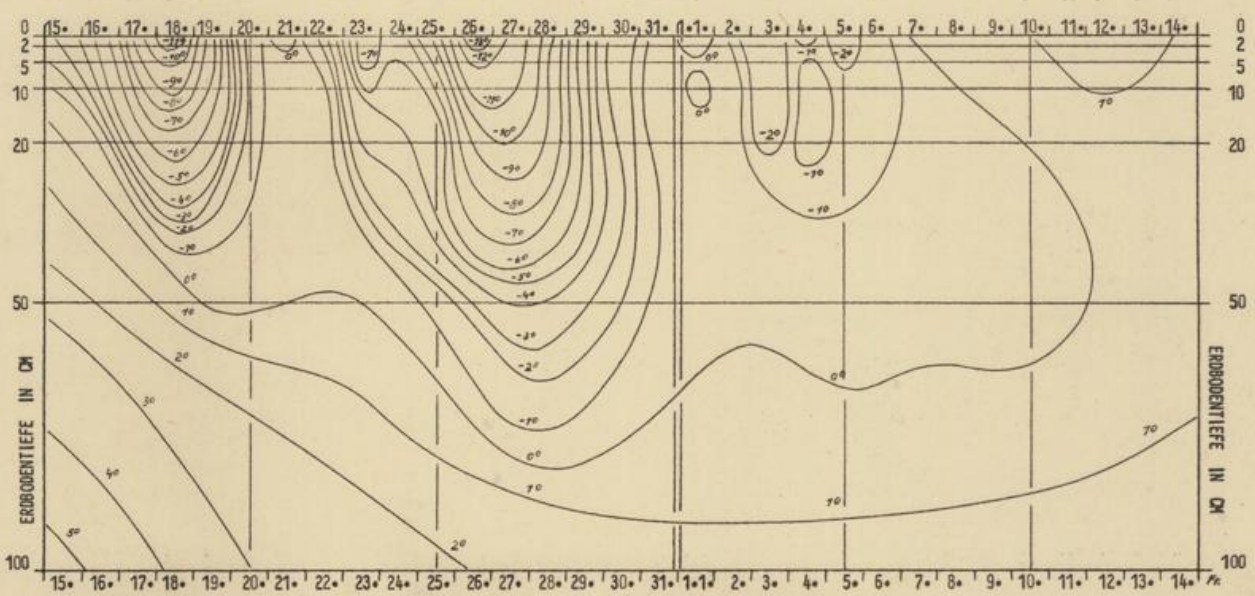
VERLAUF DER ERDBODENTEMPERATUREN IN POTSDAM FÜR DIE ZEIT VOM 15. DEZEMBER BIS 14. JANUAR 1962
