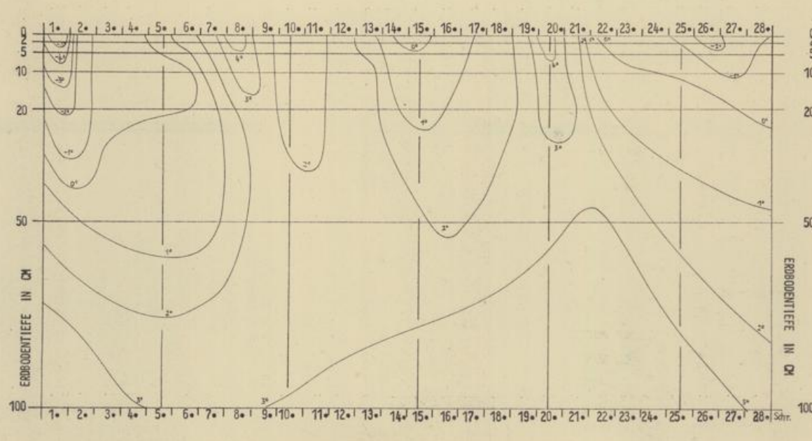
VERLAUF DER ERDBODENTEMPERATUREN IN LEIPZIG-MOCKAU IM FEBRUAR 1962
