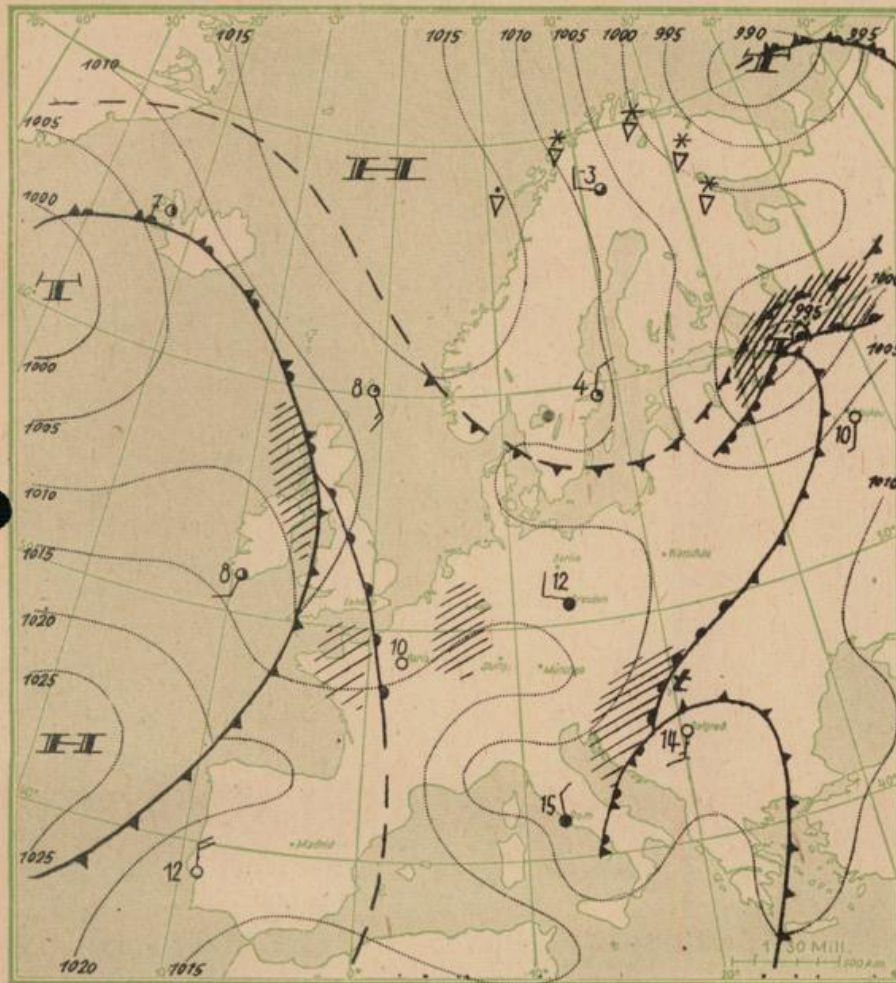
Übersichtswetterkarte 18. Mai 1947, 1 Uhr MEZ
