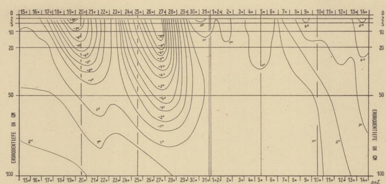
Verlauf der Erdbodentemperaturen in Potsdam in der Zeit vom 15. Januar bis 14. Februar 1961
