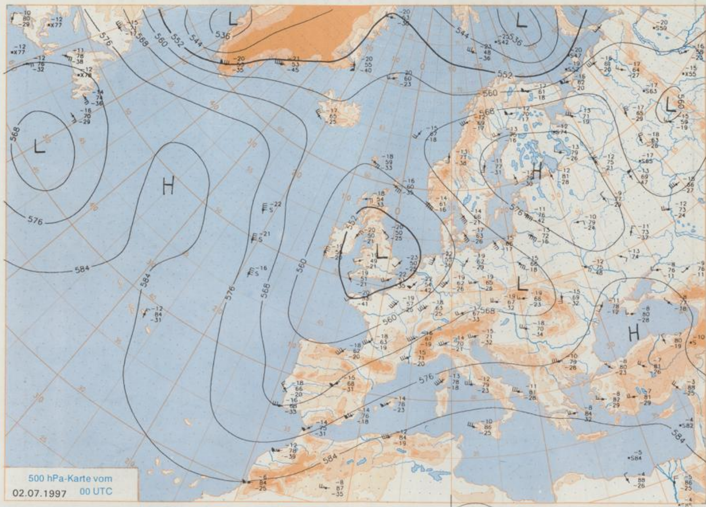
500 hPa-Karte vom 02.07.1997 00 UTC
