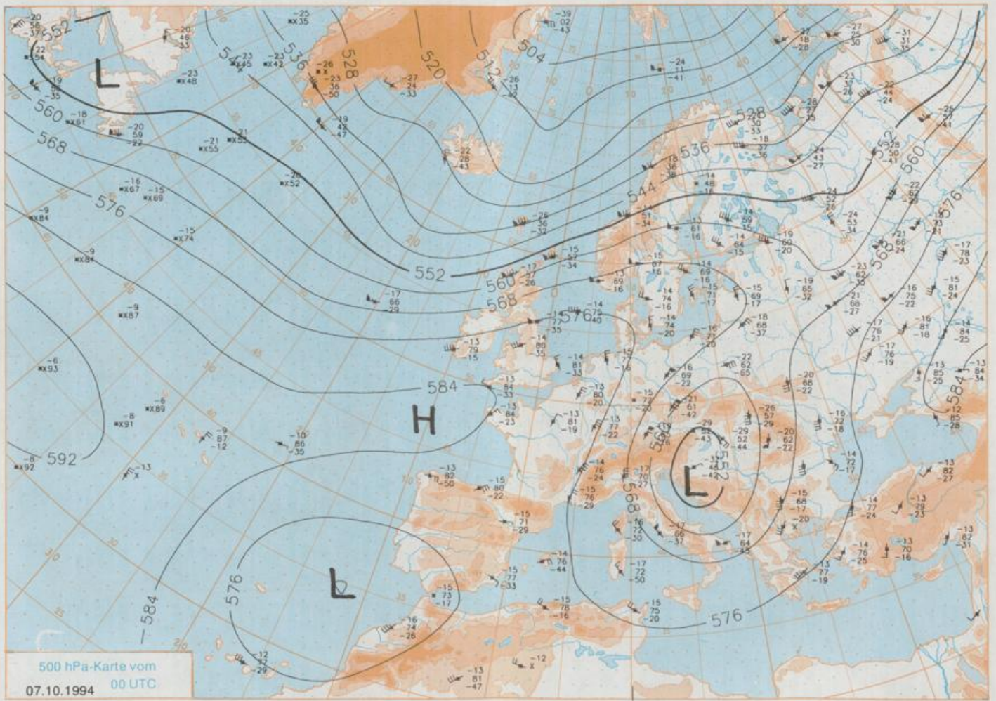
500 hPa-Karte vom 07.10.1994 00 UTC Stereographische Projektion 1 : 30 000 000 60°N
