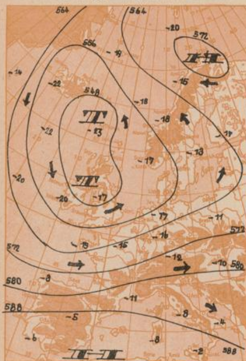
Höhenwetterkarte in ca. 5000 m Höhe (Höhenschichtlinien der 500 mb-Fläche in Dekametern) am Donnerstag, 4. August 1966 1 Uhr
