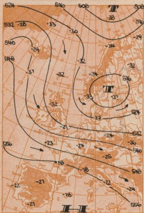
Höhenwetterkarte in ca. 5000 m Höhe (Höhensichtlinien der 500 mb-Fäche in Dekametern) am Dienstag, 1. April 1969, 1 Uhr
