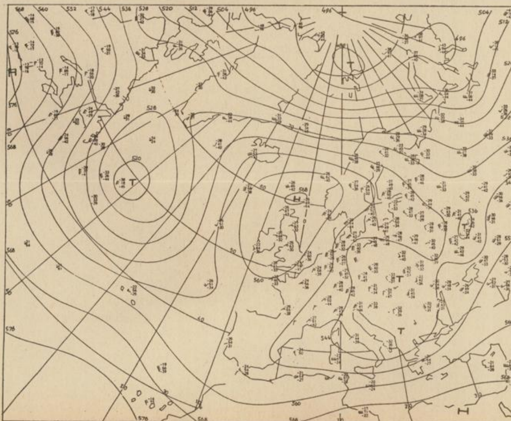
Höhenwetterkarte (Absolute Topographie 500 mb entsprechend ca. 5500 m Höhe) vom 12.3. 01 Uhr
