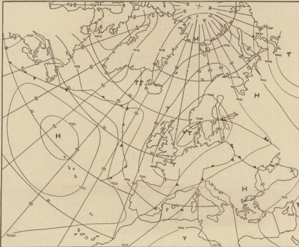
Bodenwetterkarte Vorhersage für den 18.7. 01 Uhr
