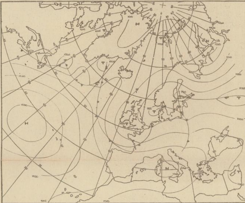
Bodenwetterkarte Vorhersage für den 21.7. 01 Uhr
