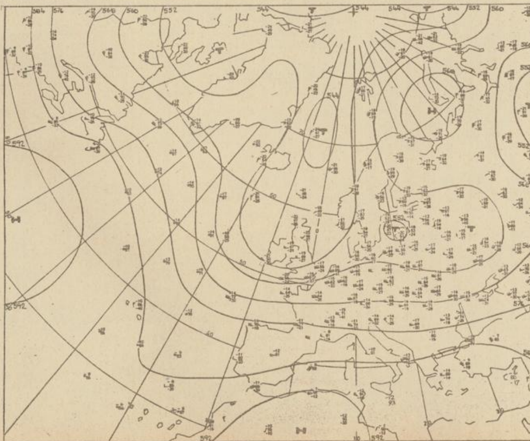
Höhenwetterkarte (Absolute Topographie 500 entsprechend ca. 5500 m Höhe) vom 20.7. 01 Uhr
