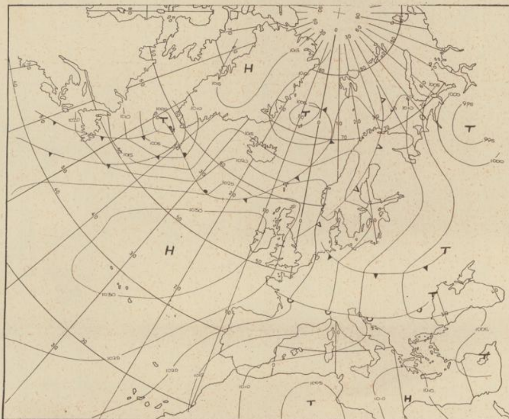
Bodenwetterkarte Vorhersage für den 30.7. 01 Uhr
