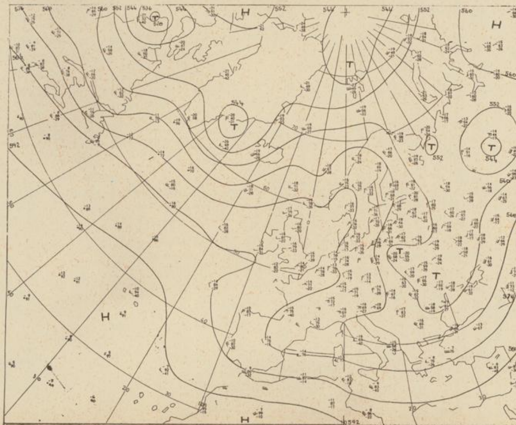
Höhenwetterkarte (Absolute Topographie 500 mb entsprechend ca. 5500 m Höhe) vom 29.7. 01 Uhr
