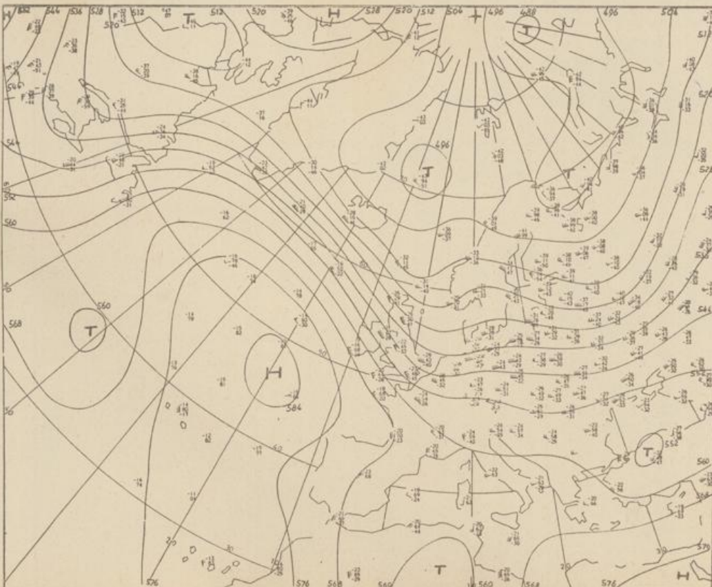
Höhenwetterkarte (Absolute Topographie 500 mb entsprechend ca. 5500 m Höhe) vom 13.12. 01 Uhr
