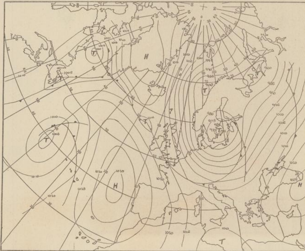
Bodenwetterkarte Vorhersage für den 14.12. 01 Uhr
