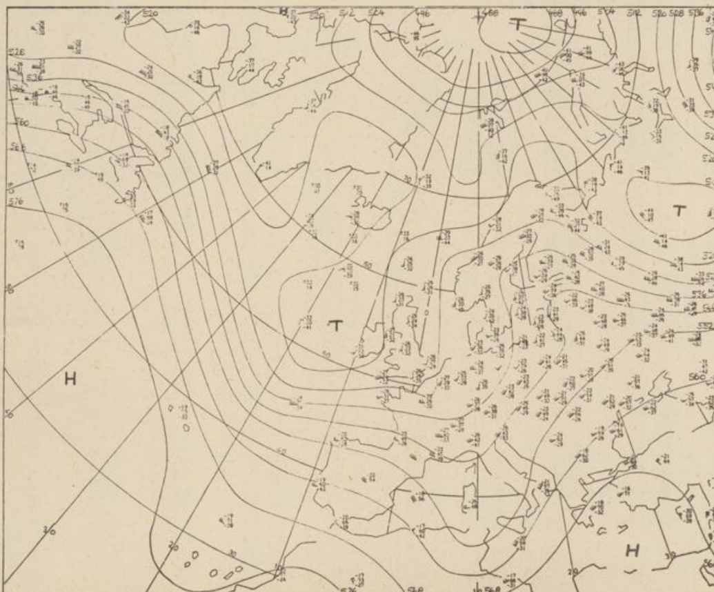
Höhenwetterkarte (Absolute Topographie 500 mb entsprechend ca. 5500 m Höhe) vom 22.12. 01 Uhr
