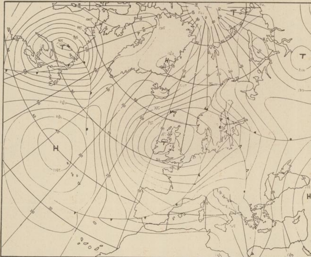
Bodenwetterkarte Vorhersage für den 23.12. 01 Uhr
