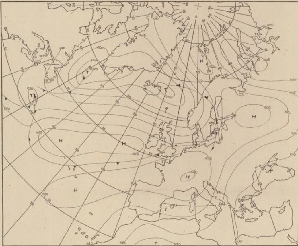
Bodenwetterkarte Vorhersage für den 3.6. 01 Uhr
