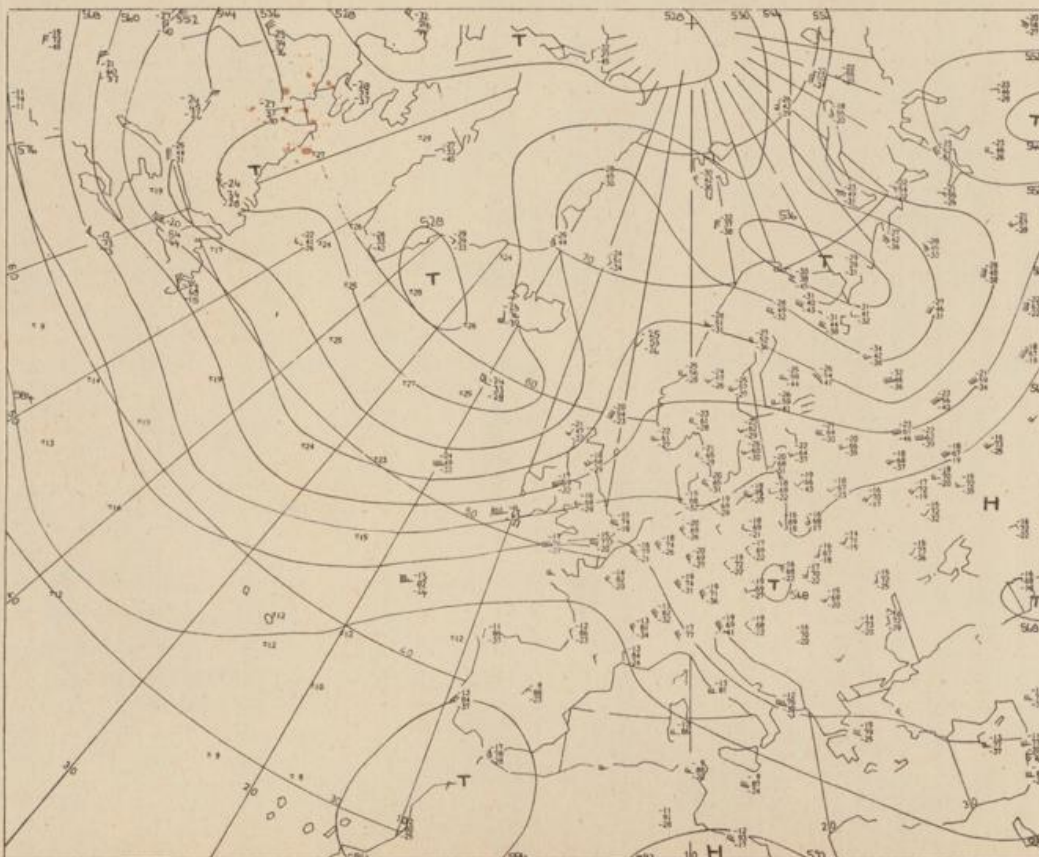
Höhenwetterkarte (Absolute Topographie 500 mb entsprechend ca. 5500 m Höhe) vom 2.6. 01 Uhr
