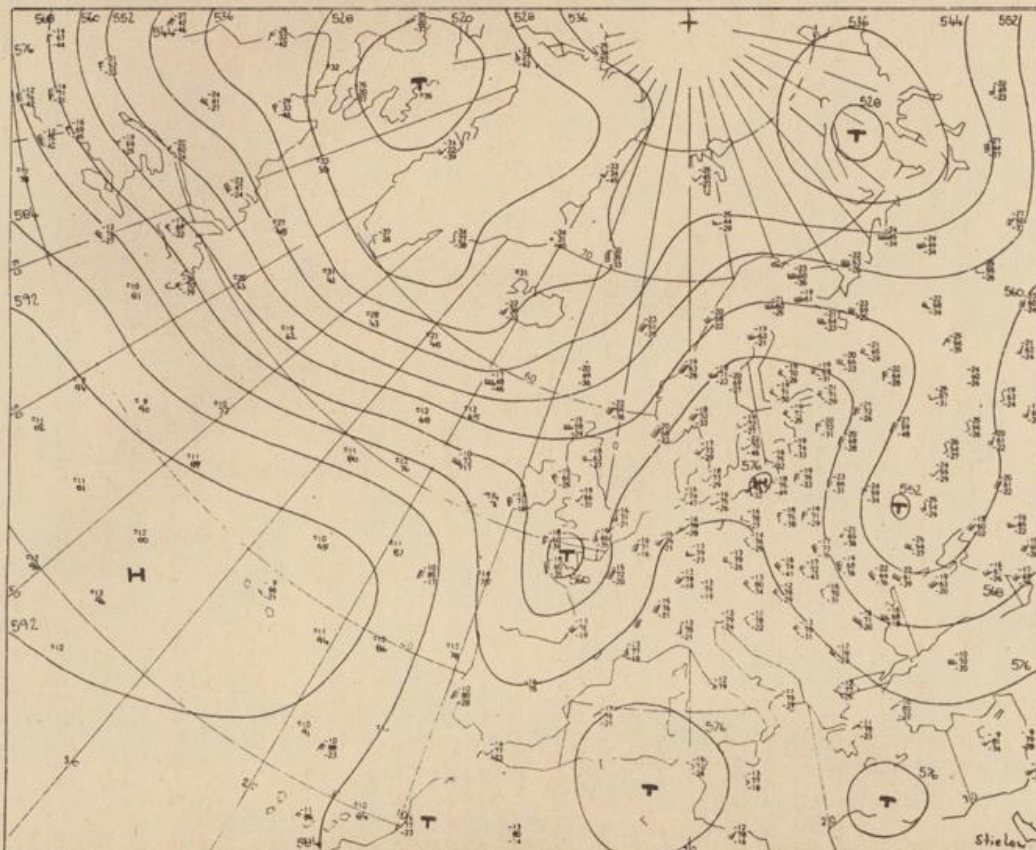
Höhenwetterkarte (Absolute Topographie 500 mb entsprechend ca. 5500 m Höhe) vom 16.9. 01 Uhr
