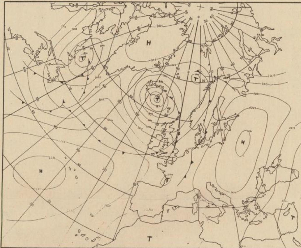
Bodenwetterkarte Vorhersage für den 17.9. 01 Uhr
