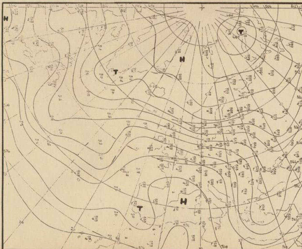
Höhenwetterkarte (Absolute Topographie 500 mb entsprechend ca. 5500 m Höhe)
