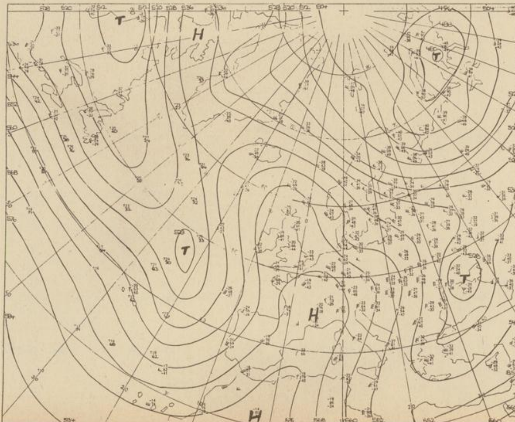
Höhenwetterkarte (Absolute Topographie 500 mb entsprechend ca. 5500 m Höhe) vom 28.2. 01 Uhr
