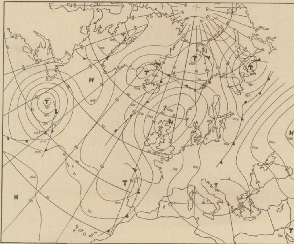
Bodenwetterkarte Vorhersage für den 17.3. 01 Uhr
