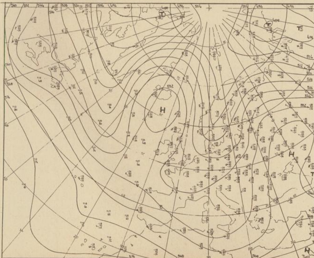
Höhenwetterkarte (Absolute Topographie 500 mb entsprechend ca. 5500 m Höhe) vom 16.3. 01 Uhr
