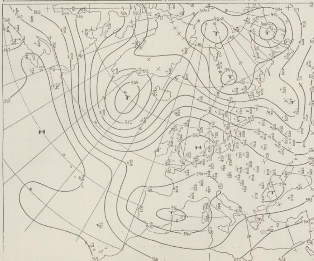
Höhenwetterkarte (Absolute Topographie 500 mb entsprechend ca. 5500 m Höhe) vom 18.01. 01 Uhr
