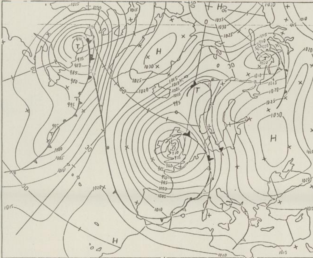
Bodenwetterkarte Vorhersage für den 22.01. 01 Uhr
