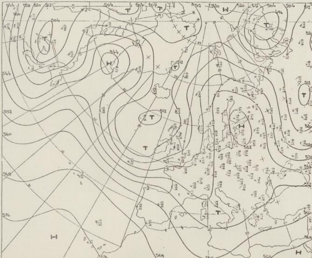
Höhenwetterkarte (Absolute Topographie 500 mb entsprechend ca. 5500 m Höhe) vom 21.01. 01 Uhr
