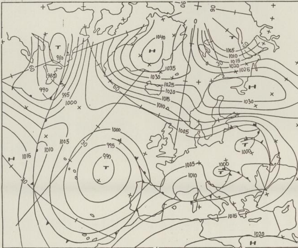
Bodenwetterkarte Vorhersage für den 25.01. 01 Uhr
