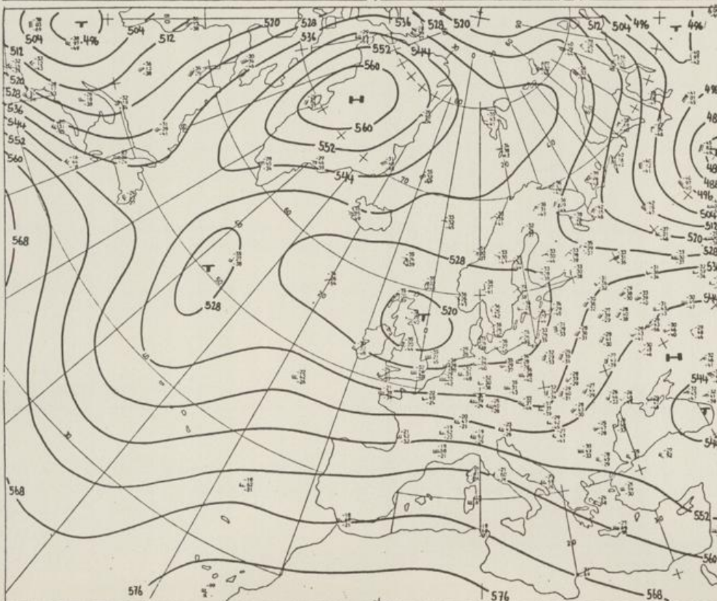
Höhenwetterkarte (Absolute Topographie 500 mb entsprechend ca. 5500 m Höhe) vom 24.01. 01 Uhr
