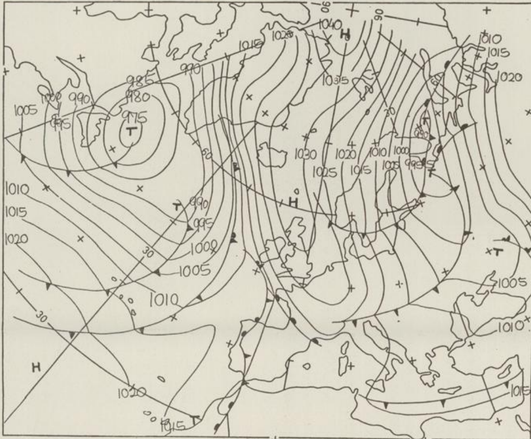
Bodenwetterkarte Vorhersage für den 27.01. 01 Uhr
