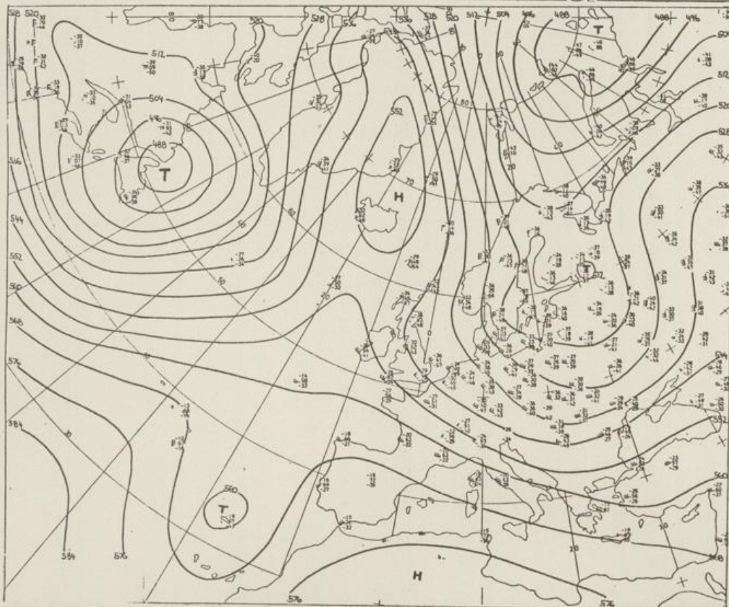
Höhenwetterkarte (Absolute Topographie 500 mb entsprechend ca. 5500 m Höhe) vom 26.01. 01 Uhr
