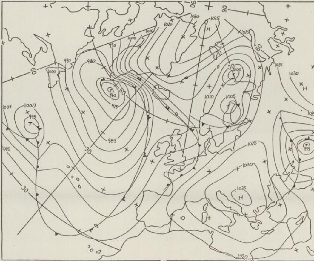
Bodenwetterkarte Vorhersage für den 29.01. 01 Uhr
