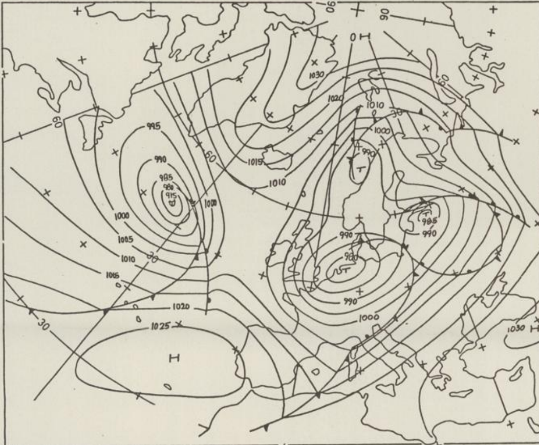
Bodenwetterkarte Vorhersage für den 01.02. 01 Uhr
