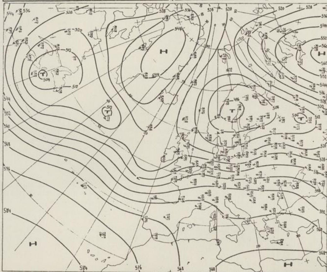
Höhenwetterkarte (Absolute Topographie 500 mb entsprechend ca. 5500 m Höhe) vom 31.01. 01 Uhr
